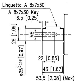
ALBERO SHAFT C25
