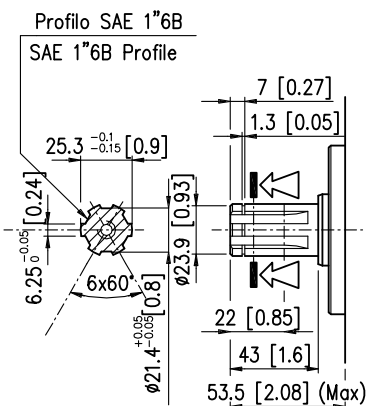
ALBERO SHAFT SD25
