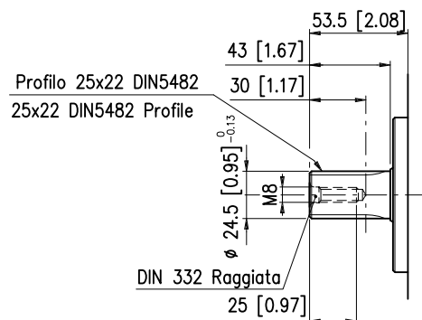
ALBERO SHAFT S 25
