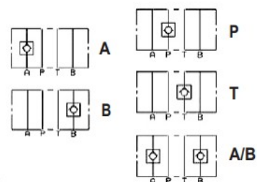
Hydraulické schéma
