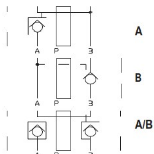
Hydraulické schéma
