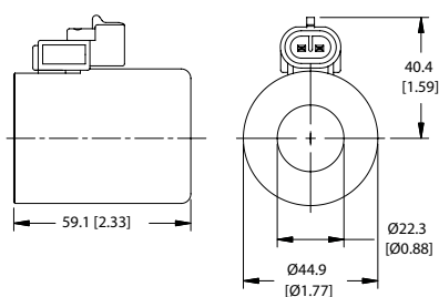
DN DIN 43650
