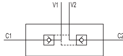
Hydraulické schéma Hydraulic diagram
